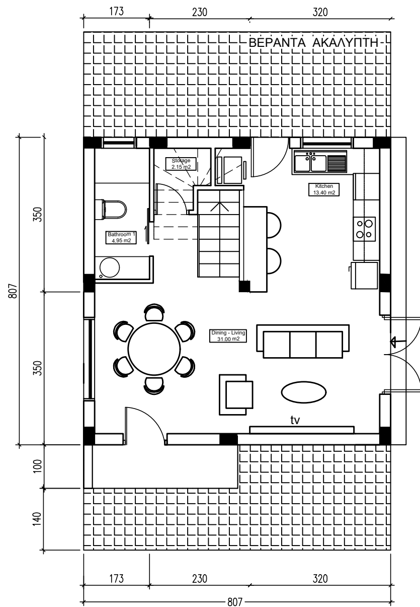
ΚΑΤΟΨΗ ΙΣΟΓΕΙΟΥ
