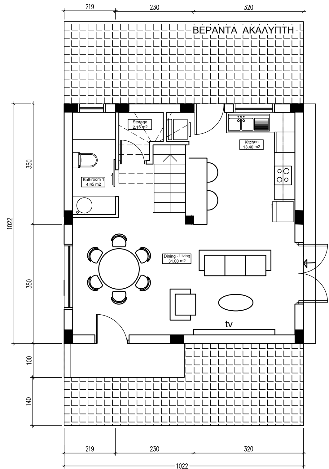
ΚΑΤΟΨΗ ΙΣΟΓΕΙΟΥ
